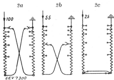
Fig. 2. Schematische Wicklungsanordnung einer regulierbaren Oerlikon-Erdschlussspule.
