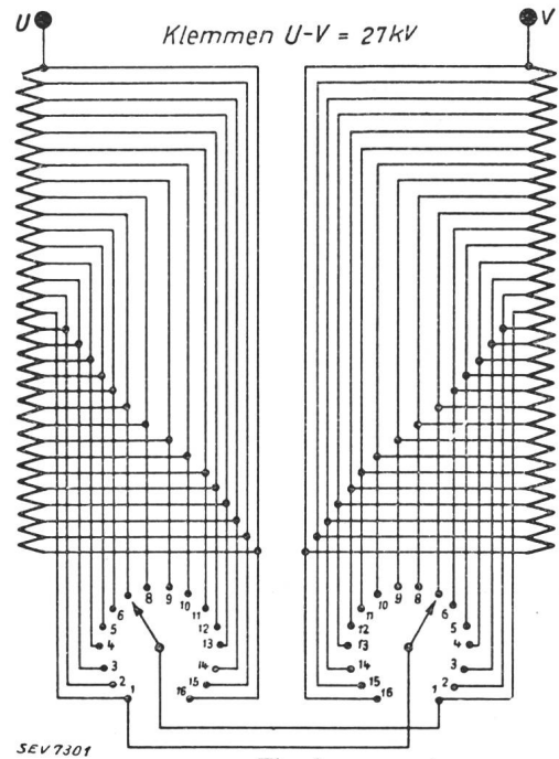
Fig. 3. Verbindungsschema einer in 16 Stufen regulierbaren Oerlikon-Erdschlussspule, mit Parallelschaltung pro Säule.
