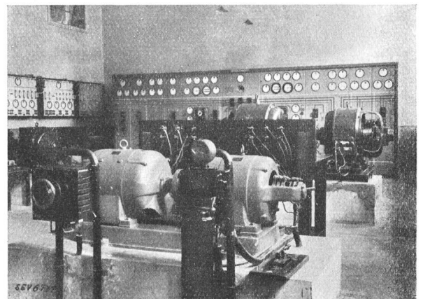
Fig. 12. Drehstromkraftwerkbetriebslaboratorium.
