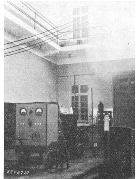
Fig. 11. Hochspannungsprüfraum mit Galerie in halber Höhe. Im Vordergrund fahrbarer 40 000-V-Prüftransformator mit Schalttafel und Induktionsregler (Brown Boveri).
