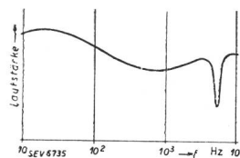
Fig. 2. Frequenzverlauf für Schallplatten- Wiedergabe bei konstanter Ein- gangs-Wechselspannung.
