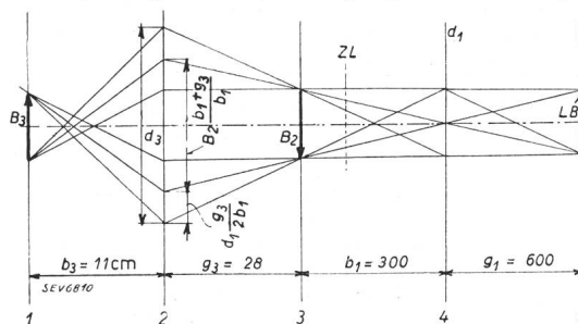
Fig. 5. Anordnung für direkten Strahlengang bei höheren Filmgeschwindigkeiten.
