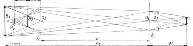
Fig. 2. Strahlengang.
