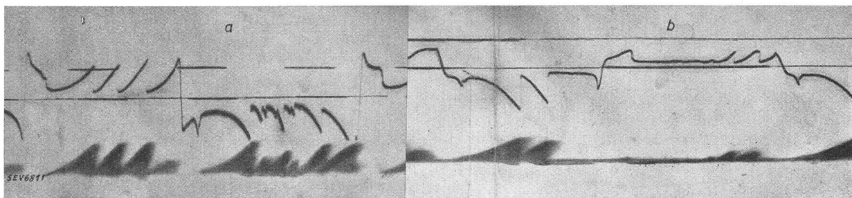
Fig. 4. Lichtbogaufnahmen, Oszillogramme in 1/2 der natürlichen Grösse.
