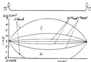
Variation de la pression p pendant l'échauffement par différentes charges et le refroidissement d'un câble à huile de grande longueur, compensé à ses extrémités seulement.
