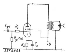
Fig. 4. Normale Schaltung der AL5 als Leistungsverstärker.
