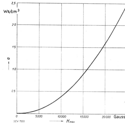
Fig. 3. Kurve der einmaligen Magnetisierungsarbeit von 0 bis H_{max} pro \text{cm}^3 Luft, für verschiedene Werte von H_{max} , abgeleitet aus der Formel
