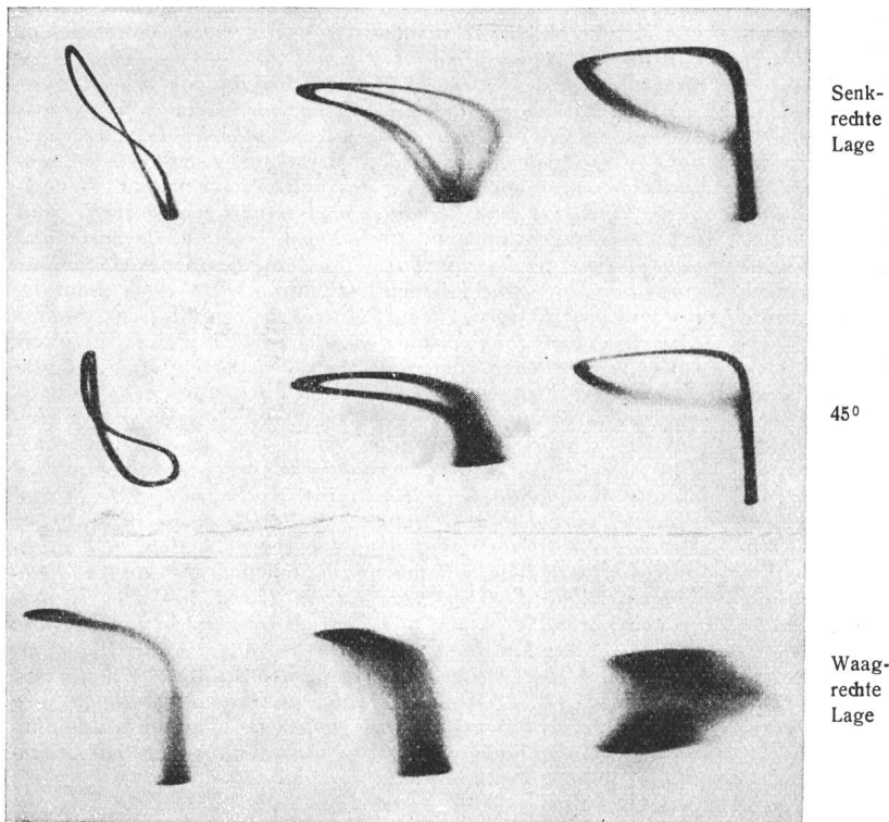
Fig. 1. Kennlinien eines Fernsprechmikrophons.
