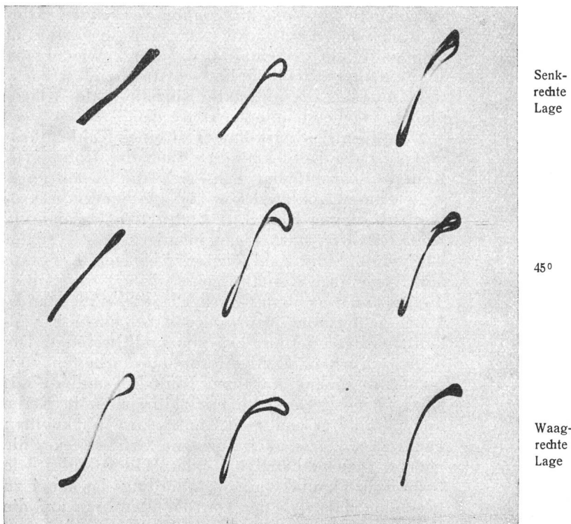
Fig. 2. Kennlinien eines Stern-Elektrodenmikrophons.
