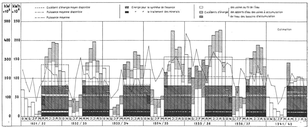
Fig. 3. Variation des excédents d'énergie mensuels et des puissances utilisables de 1931/32 à 1936/37 et 1941/42.
