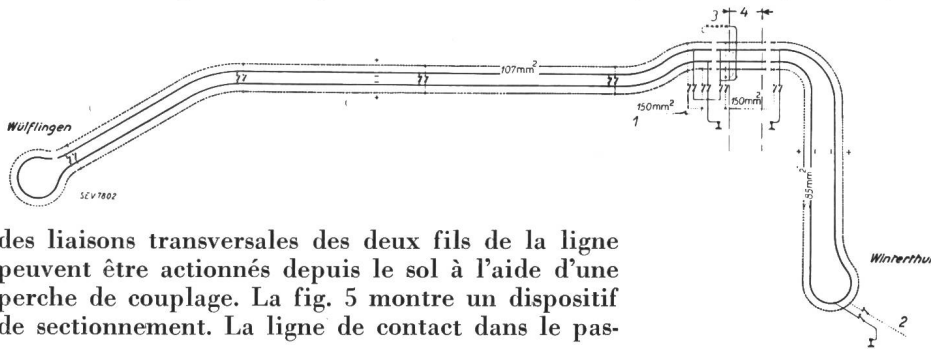
Fig. 4. Ligne de contact Winterthur gare CFF - Wülflingen. Schéma de couplage. 1 Feeder du réseau de distribu- tion communal. 2 Ligne de contact du tramway. 3 Lampes de signalisation. 4 Passage sous voies.
