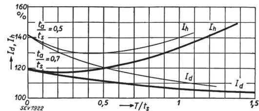
Fig. 4. Courant nécessaire en régimes continu et unihoraire en fonction des constantes de temps relatives T/t_s pour deux valeurs constantes de t_a/t_s (0,5 et 0,7) la moyenne des carrés du courant étant égale à 100 %.
