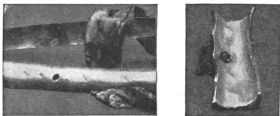
Fig. 2. Beispiele von Blitzschäden an Bleimänteln.
