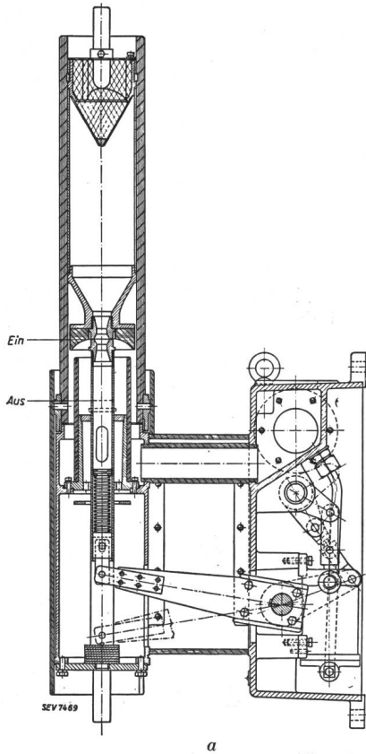
Fig. 14. Druckluftschalter mit Doppeldüse ohne (links) und mit Widerstandsstufe (rechts). W Widerstand. K Widerstandskontakt.
