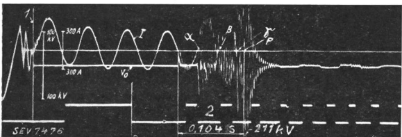
Fig. 18. Abschaltung eines Kurzschlusses hinter einer langen 132-kV-Leitung.
