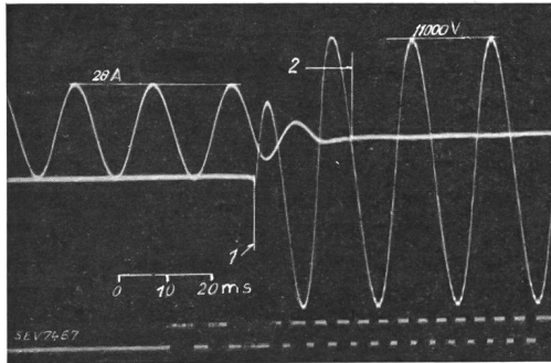
Fig. 12. Schleifenoszillogramm einer Widerstandsabschaltung mit einem Wasserschalter (Typ WS 46.6, 10 kV, 600 A). 1 Beginn der Öffnung der Kontakte 2 Ende der Abschaltung.
