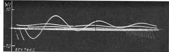
Fig. 7. Rückzündungen.
