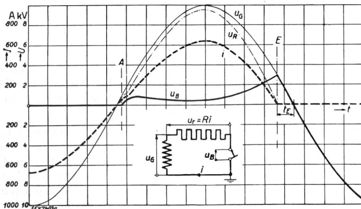
Fig. 8. Prinzipieller Verlauf einer Wechselstrom-Abschaltung bei \cos \varphi = 1 .
