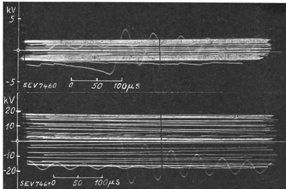
Fig. 6. Einwirkung der Lichtbogenlöscheinrichtung auf die wiederkehrende Spannung.
