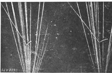
Fig. 6. Wilsonaufnahme der Stickstoffzertrümmerung durch He-Kerne. Die sich quer durch das Strahlenbüschel ziehende Spur rührt von einem bei der Umwandlung emittierten Proton her.
