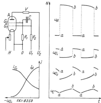
Fig. 2. Kippschaltung mit einer Doppelgitterröhre. V Verbraucher.
