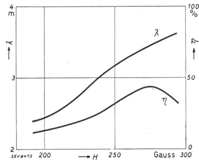
Fig. 8. Wellenlänge und Wirkungsgrad in Funktion der Feld- stärke beim 2-Oszillo- den-Magnetron.
