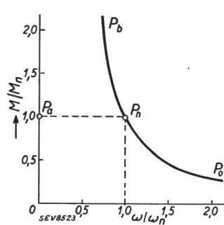
Fig. 3. Idealer Gleichstrom-Reihenschlussmotor.
