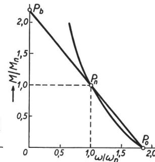
Fig. 4. Allgemeine Idealturbine.
