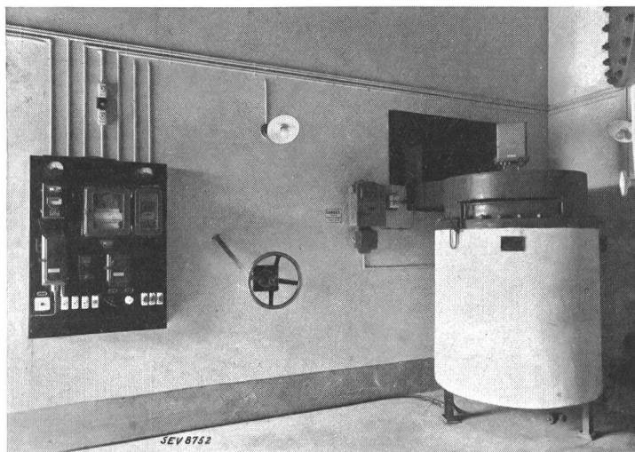
Fig. 3. Intérieur de la chaufferie.
