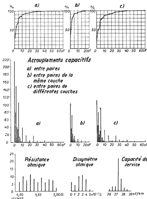
Fig. 4. Câble téléphonique, 40 paires 1,3 mm \varnothing , conducteurs en aluminium. Abcisses: valeurs mesurées. Ordonnées: nombres de valeurs correspondantes.
