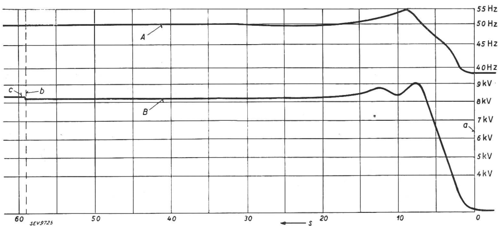
Fig. 2. Reguliertvorgang beim Parallelschalten mit elektrischem Primärregler. A Einschwingen der Frequenz. B Einschwingen der Spannung. a Einschalten des Spannungsreglers. b Parallelschaltmoment. c Netzspannung.
