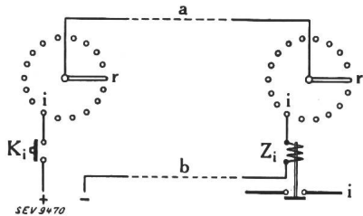
Fig. 3. Grundätzliche Anordnung einer Fernsteuer-Einrichtung mit einfacher Umschaltung der Uebertragungsleitung
