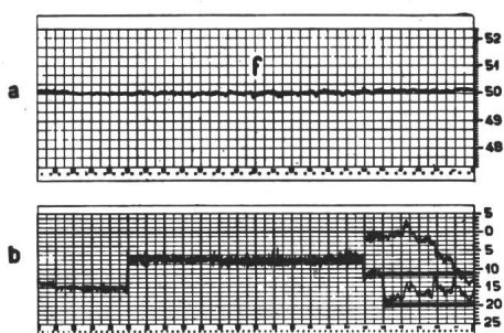
Fig. 4. Uebergabeleistung (Handregulierung). + bedeutet Lieferung - bedeutet Bezug
