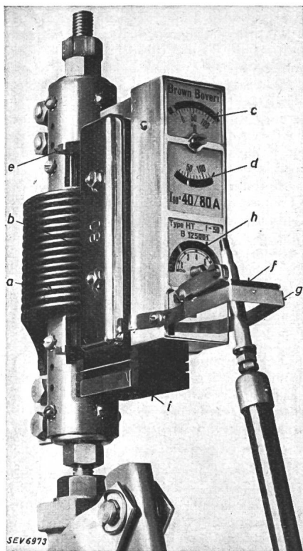
Fig. 9. Hauptstromthermorelais Typ HT. a Stromspule b Wärmeträger c Anzeige der Uebertemperatur d Einstellskala der Auslöse-Uebertemperatur e Keile zur Strom- bzw. Temperatureinstellung f Auslösehebel g Auslösesignal h Grenzstrom-Auslösung i Kompensation der Umgebungstemperatur
