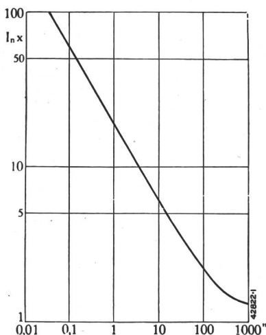
Fig. 1. Charakteristischer Verlauf der Strombelastbarkeit eines Leiters in Abhängigkeit von der Zeit («Gefahrenlinie»).
