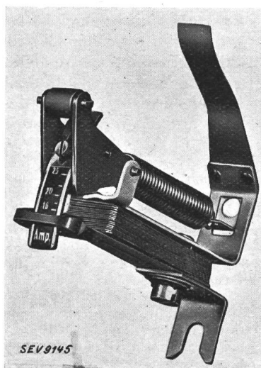
Fig. 2. Direkt beheizter Paketwärmeauslöser mit Kraftspeicher.
