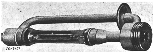
Wassergekühlte Höchstdruck-Quecksilberdampf Lampe (oben) mit einem Lichtstrom von 120 000 Lumen, Leistungsaufnahme 2300 W, einschliesslich Vorschaltgerät. Praktische Anwendung (links) der oben dargestellten Lampe in einem Landebahnscheinwerfer mit angebautem Kühlaggregat.
