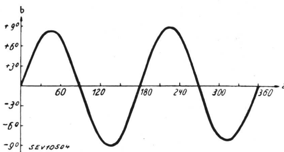
Fig. 6. Funkbeschiebungskurve
