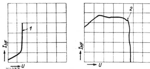
Fig. 8. Vergleich der Steuerkurven von Turbator (oben) und Magnetron (unten)
