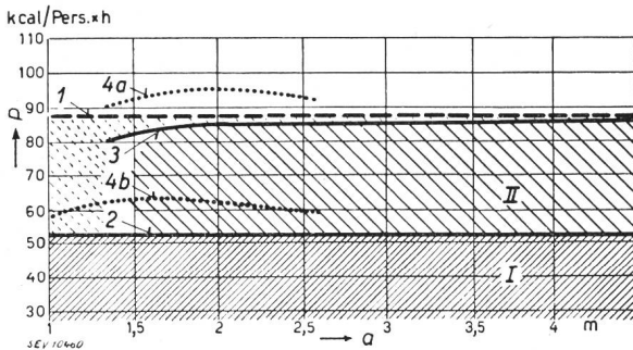
Fig. 3a. Konvektionsöfen
