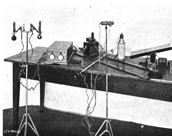
Fig. 2. Elektrische Messausrüstung.
