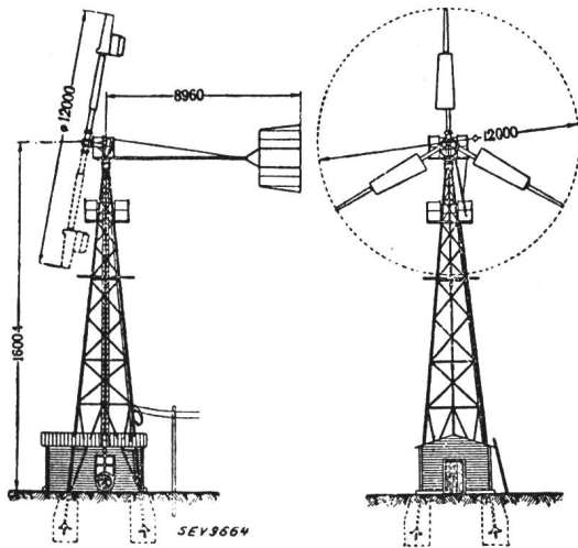
Fig. 1. Windmotor WIME-D 12.
