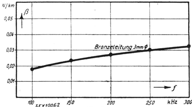
Hochfrequenz-Dämpfung einer 3-mm-Bronze-Freileitung.
