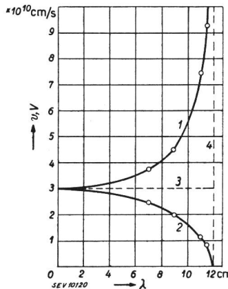
Fig. 4. Frequenzgang von Phasen- und Gruppengeschwindigkeit. Kurven errechnet, Punkte gemessen. 1 Phasengeschwindigkeit V , 2 Gruppengeschwindigkeit v , 3 Lichtgeschwindigkeit c , 4 Grenzwellenlänge.
