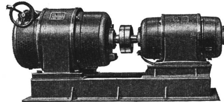
Umformergruppe, bestehend aus: Drehstrom-Nebenschluss-Kommutatormotor 500...2000 U./min, regulierbar, gekuppelt mit Einphasen-Synchron-Generator mit variabler Frequenz 50...200 Hz.
