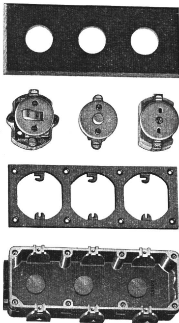
Links: Gardy U.P.-Apparate-Zusammenbausystem für Selbstkombination.
