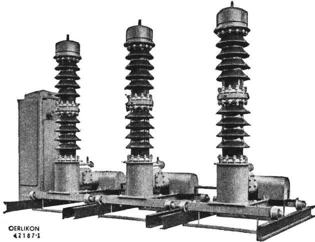
Fig. 4. Oelarmar Schnellschalter 64 kV, 600 000 kVA.
