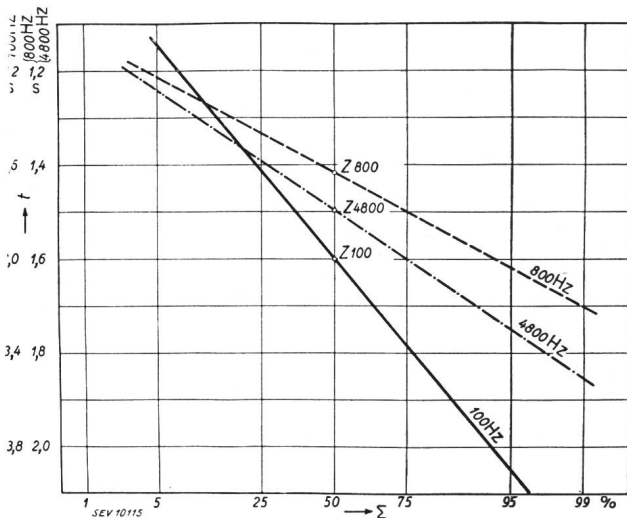
Fig. 8. Merkmalsgrenzwert (Nachhallzeit) t (in s) in Funktion der Summenhäufigkeit \Sigma (in %) Studio Basel (1).
