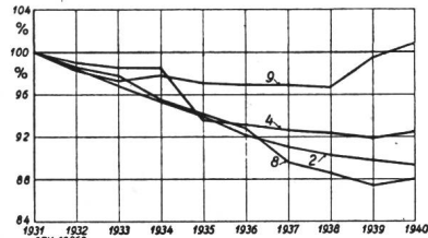
Fig. 3. Entwicklung des mittleren Anschluss- wertes pro Apparat 1931...1940 (1931 = 100).
