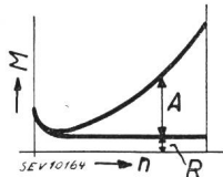
Fig. 1c. Von der Drehzahl gesetzmässig abhängiges Arbeitsdrehmoment.
