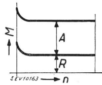
Fig. 1b. Gleichbleibendes, von der Drehzahl unabhängiges Arbeits-Drehmoment.
