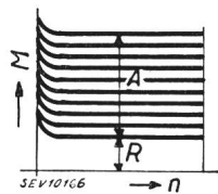
Fig. 1e. Willkürlich und unabhängig von der Drehzahl veränderliches Drehmoment.
