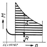
Fig. 1f. Willkürlich veränderliches, aber in seiner Grösse an die Drehzahl gebundenes Arbeitsdrehmoment.
