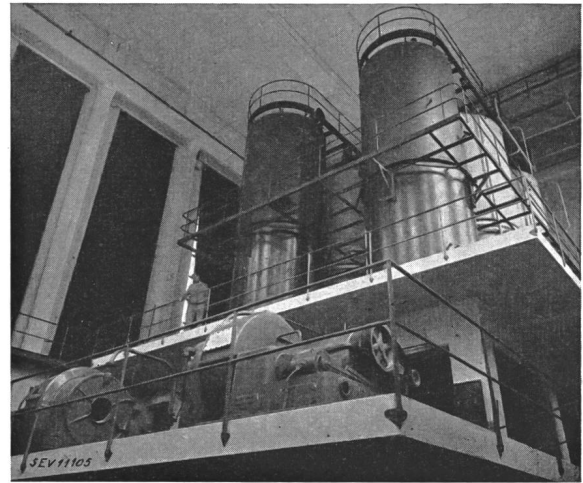
Fig. 6. Evaporateurs et, au premier plan, essoreuses à débit continu (Nos. 5 et 12 du schéma).
