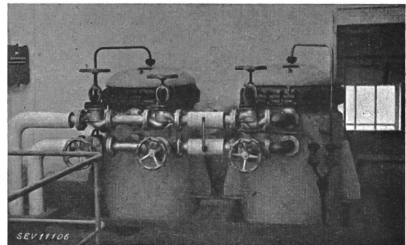
Fig. 7. Réchauffeur pour la saumure (No. 4 du schéma).
