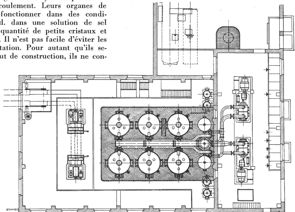
Fig. 4. Disposition générale de l'installation. Plan.
