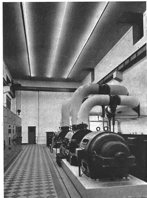
Fig. 1. Kompressorenhalle Ryburg.
