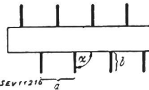
Fig. 5. Schematische Darstellung von Widerständen mit normaler Wendelanordnung (oben) und solche mit radialer Stellung der Wendel (unten)
