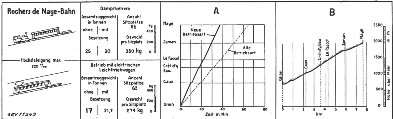
Fig. 6. Zahnradbahn Glion-Rochers de Naye Zuggewicht, Sitzplätze und Fahrzeiten beim Dampfbetrieb und beim elektrischen Betrieb. A Graphischer Fahrplan. B Längenprofil.
