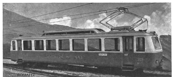
Fig. 7. Leichttriebwagen der Zahnradbahn Glion-Rochers de Naye Spurweite 800 mm. Zahnstange Abt. Maximalsteigung auf der Zahnstangenstrecke 220 ‰. (Mech. Teil: SLM, Winterthur; Elektr. Teil: Brown, Boveri)
