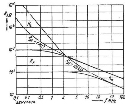
Fig. 3. Wirkwiderstände eines 1-M \Omega - und eines 100-k \Omega -Widerstandes (Index L deutet auf ungeerdeten, Index K auf geerdeten Widerstand)
