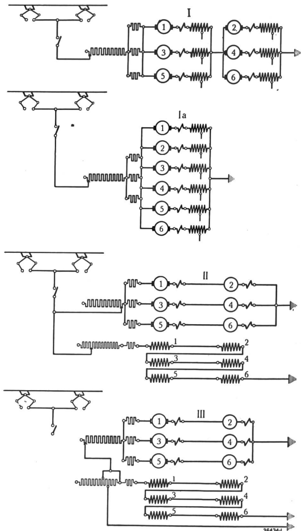
Fig. 5. Grundsätzliches Schaltbild der verschiedenen Motorengruppierungen der MOB-Lokomotive von Fig. 4
