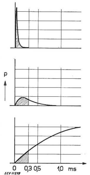
Fig. 18. Schalldruckverlauf von 3 Einzelknacken der gleichen Lautstärke von 65 phon Nur die ersten 0,3 ms (schraffierte Flächen) sind für die empfundene Lautstärke massgebend, der spätere Verlauf ist belanglos. (Nach Steudel.)
