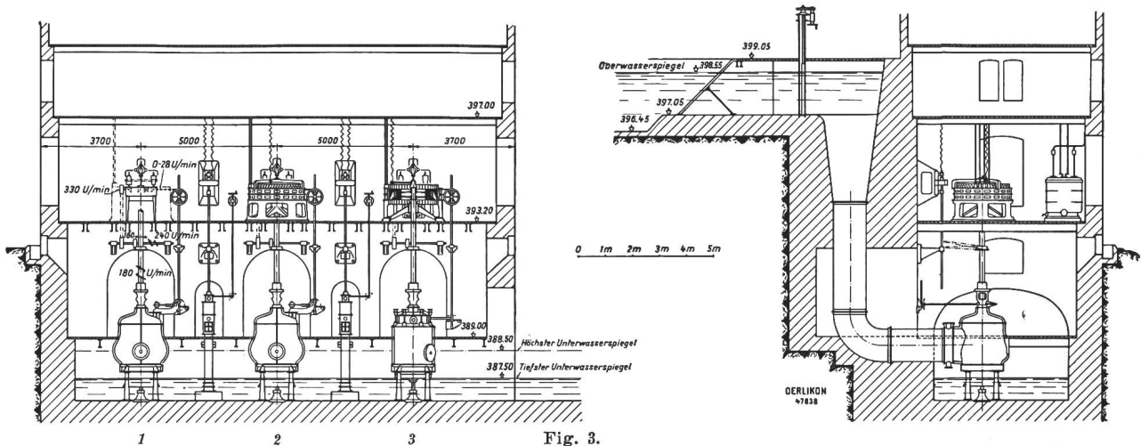
Fig. 3. Kraftwerk Hochfelden vor dem Umbau 1, 2 Francisturbinen aus dem Jahre 1903. 3 Jonvalturbine aus dem Jahre 1892.
