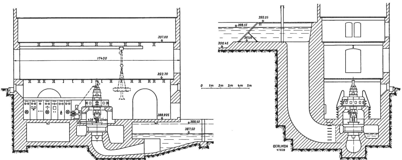
Fig. 4. Kraftwerk Hochfelden nach dem Umbau im Jahre 1942 Eine Kaplan-turbine 540 kW mit zugehörigem Generator 620 kVA, 380/220 V, 50 Hz
