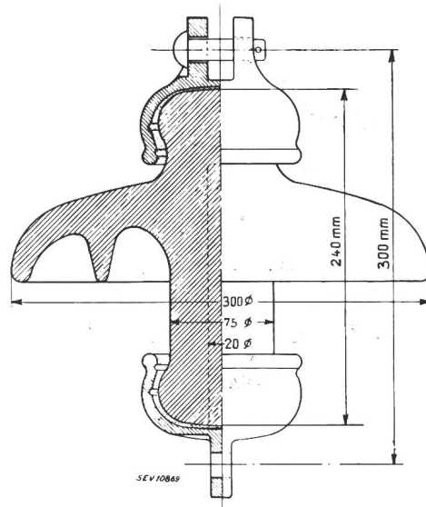
Fig. 1. Erster in der Praxis verwendeter 50-kV-Motor-Isolator (Fabrikation 1918)
