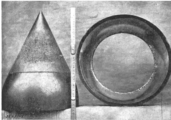
Fig. 1. Abgenutzte Nadel mit zugehörigem Düsenring Tiefe der Erosionsrinnen: 0,5...1 mm. Material: Stahlguss, unlegiert. Benutzungsdauer: 8200 Betriebsstunden.
