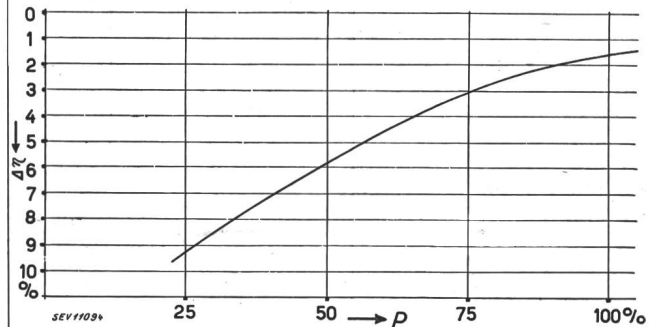
Fig. 4. Verminderung des Wirkungsgrades der Turbine \Delta\eta verursacht durch die Abnutzung der Nadeln und Düsen, in Abhängigkeit der Turbinenbelastung P .
