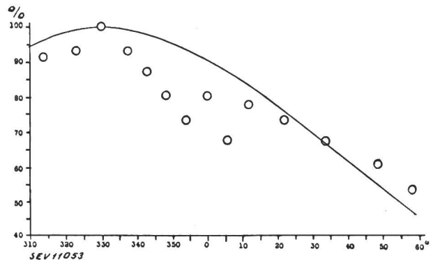
Fig. 17. Strahlungsintensität als Funktion der galaktischen Länge Ordinate: Intensität in Prozenten der Maximalintensität. Abszisse: Galaktische Länge in Grad.
