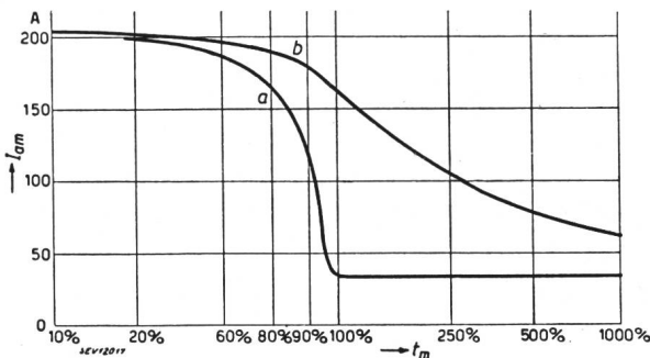
Fig. 2. Motor-Anlaufcharakteristik
