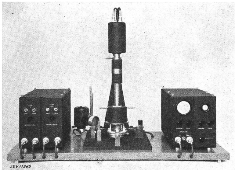
Fig. 1. Auswuchtgerät für Kreisel
