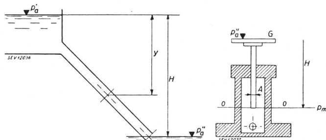
Fig. 1. Definitions-Skizze für Gefälle und Drücke
