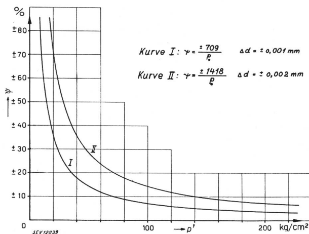
Fig. 4. \psi -Werte in Funktion der Pressung p' , d. h. des Gefälles H
