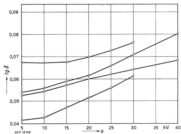
Fig. 4. Dielektrische Verluste ( \text{tg}\delta ) von Statorspulen verschiedenen Fabrikates in Funktion des Effektivwertes der Spannung ( U )
