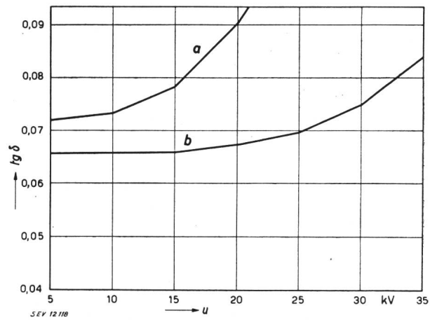
Fig. 3. Dielektrische Verluste ( \text{tg}\delta ) in Funktion des Effektivwertes der Spannung ( U )
