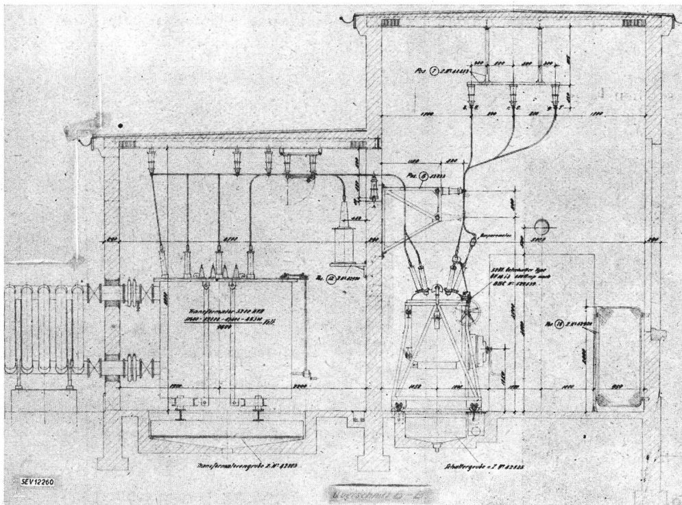
Fig. 2. 3,2-MVA-Transformator 50/10 kV Innenaufstellung auf schallisoliertem Fundament, Kühler im Freien; natürlicher Oelumlaufl und natürliche Kühlung.
