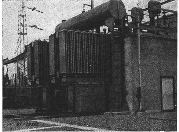
Fig. 7. 35-MVA-Transformator 150/80/50 kV mit natürlichem Öelumlaufl und forcierter Luftkühlung. Transformator in schalldichter Umbauung. Kühler im Freien.
