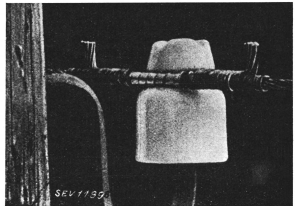
Fig. 16. Beugli constitué par un tronçon de câble Vue de l'arrière.
