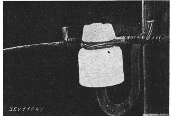
Fig. 15. Beugli constitué par un tronçon de câble Vue de face.
