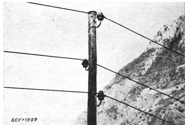
Fig. 17. Ligne de montagne en alliage Ad avec beuglis Beugli en aluminium massif profilé. Noter la distance relativement grande qui sépare les conducteurs et qui est motivée par les grandes portées (plus de 50 m) rendues nécessaires en raison de la configuration du terrain.
