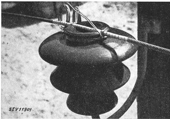
Fig. 19. Confection d'une attache sur la tête d'un isolateur prévu spécialement dans ce but
