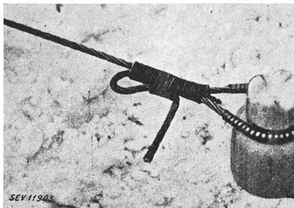
Fig. 22. Attache terminale ou d'arrêt prévue pour dérivation. Noter la boucle allongée que forme le câble.
