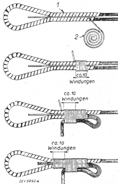
Fig. 21. Attache terminale 1 Ruban en aluminium recuit de 10·1 mm; pour des conducteurs minces un ruban plus étroit peut même être préférable. 2 Fil de ligature en aluminium recuit de 2,5 à 4 mm Ø. Pour les conducteurs massifs, il n'est pas nécessaire de recourber complètement et de ligaturer l'extrémité du conducteur; il suffit de la redresser.
