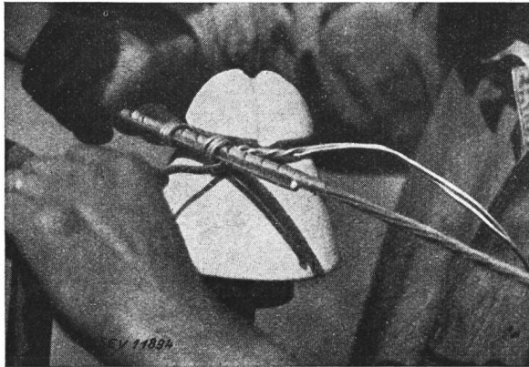
Fig. 12. Confection d'une attache croisée avec deux fils de ligature. Remarquer combien le fil de ligature entourant le conducteur est rapproché de la gorge de l'isolateur!
