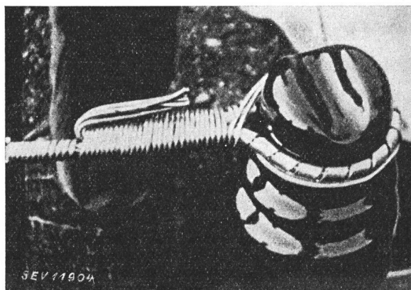
Fig. 23. Attache terminale incorrecte Le câble est trop étroitement cintré autour de la gorge de l'isolateur.
