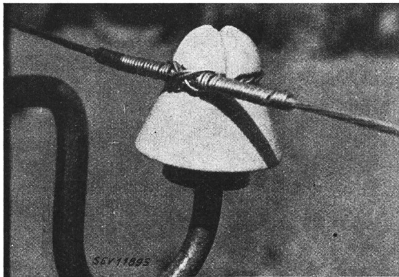
Fig. 13. Attache croisée avec deux fils de ligature
