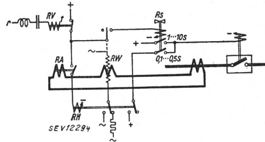
Fig. 5. Einpolig dargestellte Entkopplungseinrichtung
