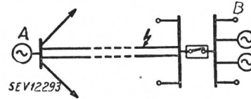
Fig. 4. Störung durch Kurzschluss im Fremdnetz
