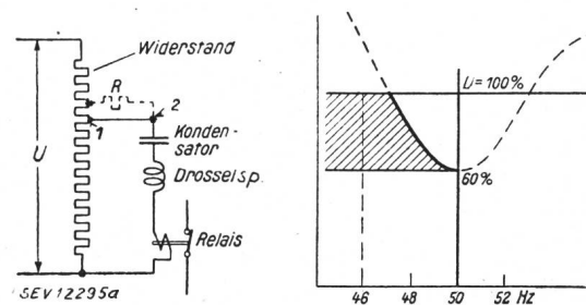
Fig. 6. Frequenzabhängiges Spannungsrelais Schaltung von R siehe Text. Ansprechverlauf des Spannungsrelais
