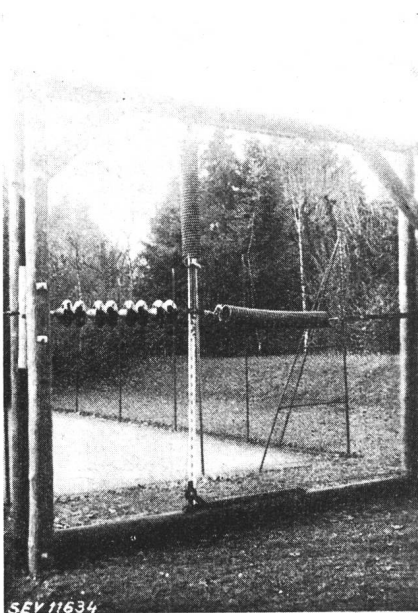
Fig. 7. Isolatoren-Prüf-Einrichtung für dynamische Beanspruchung der Prüfobjekte Beide Zugfedern entspannt
